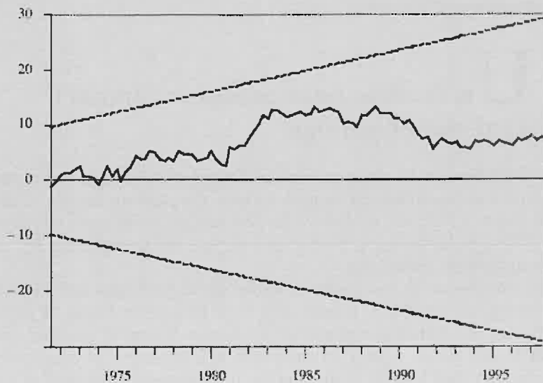
Test de stabilité Cusum au seuil de 5 %
