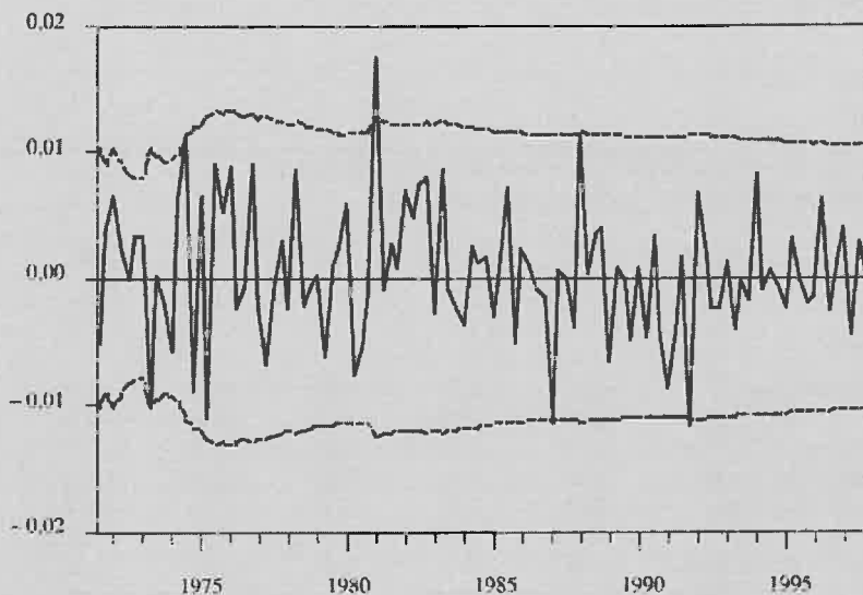
Test de stabilité des résidus récursifs
